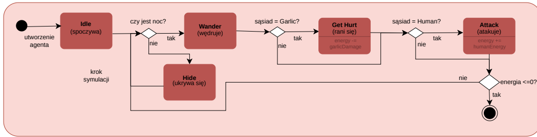
DIAGRAM STANÓW -- AGENT (PRZYKŁADY)
