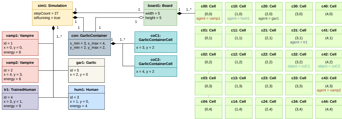
DIAGRAM OBIEKTÓW (PRZYKŁADOWA INSTANCJA)
